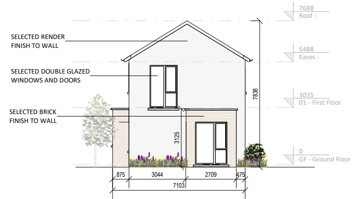
7 H03B Right Elevation 1 : 200
