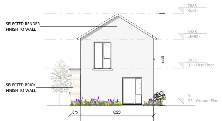
5 H03R Right Elevation 1 : 200
